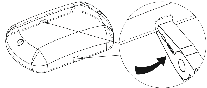
Рисунок 3 — Расположение выламываемых вставок в корпусе светильника СА-5006Д
