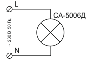
Рисунок 2 — Схема подключения светильника СА-5006Д
